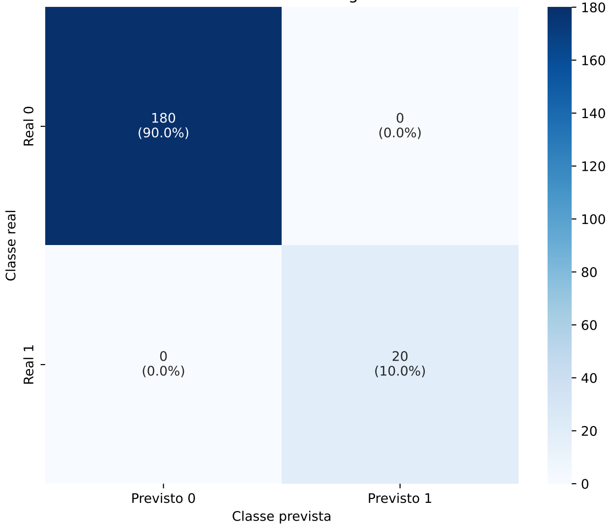
Matriz de Confusão — xgboost
